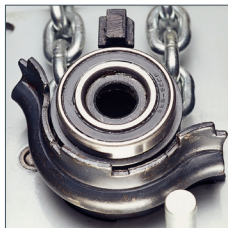
Chain guide
